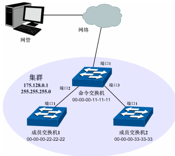
图 14-19 集群管理组网图
