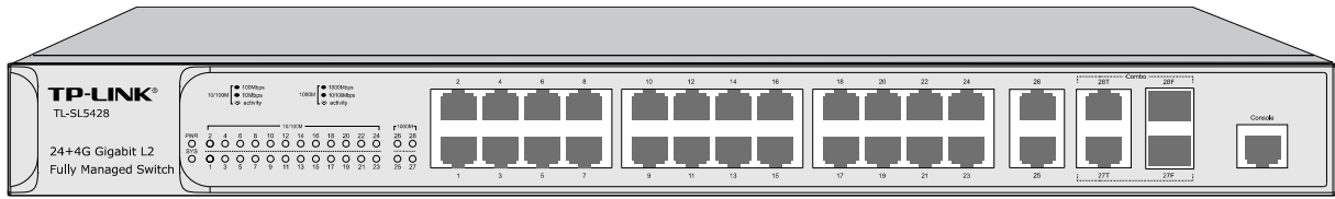
图 2-1 前面板
