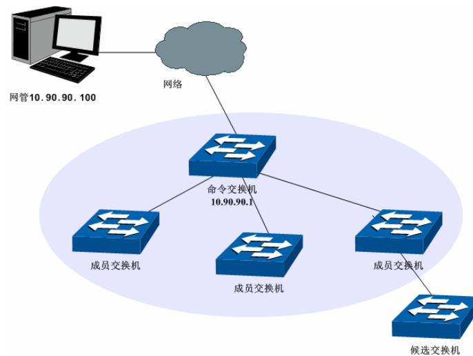
图 14-1 集群典型应用组网图
